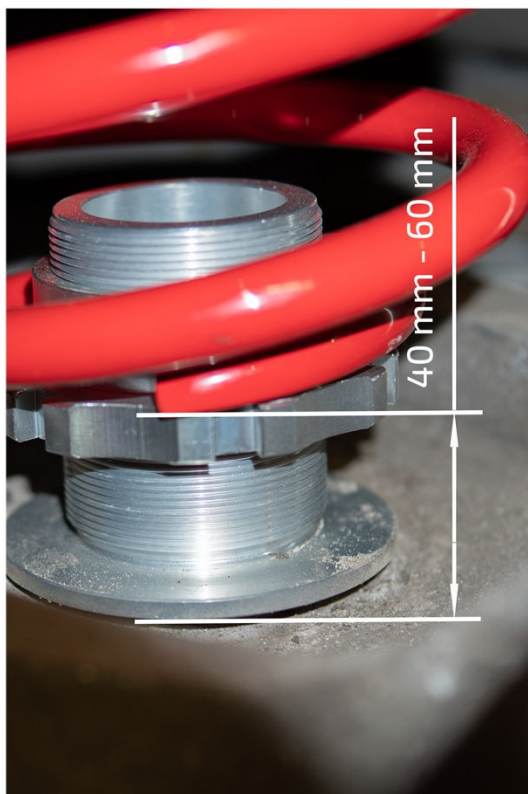
Hinterachse
