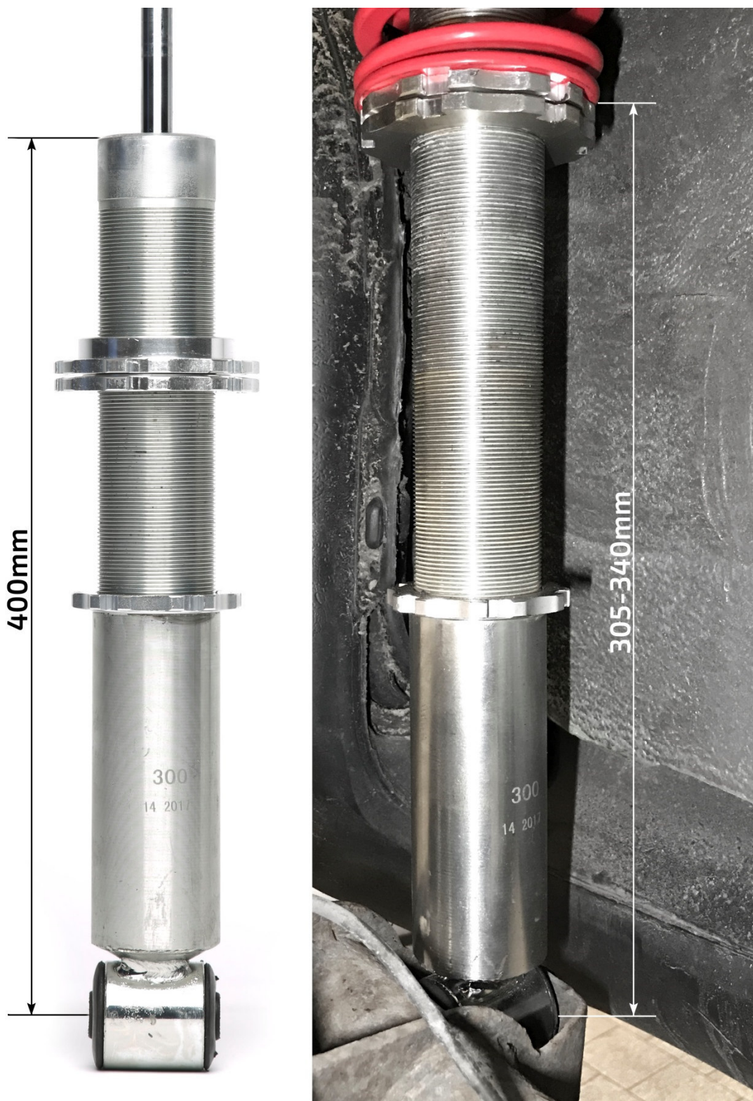
Fahrwerk Achse 2
