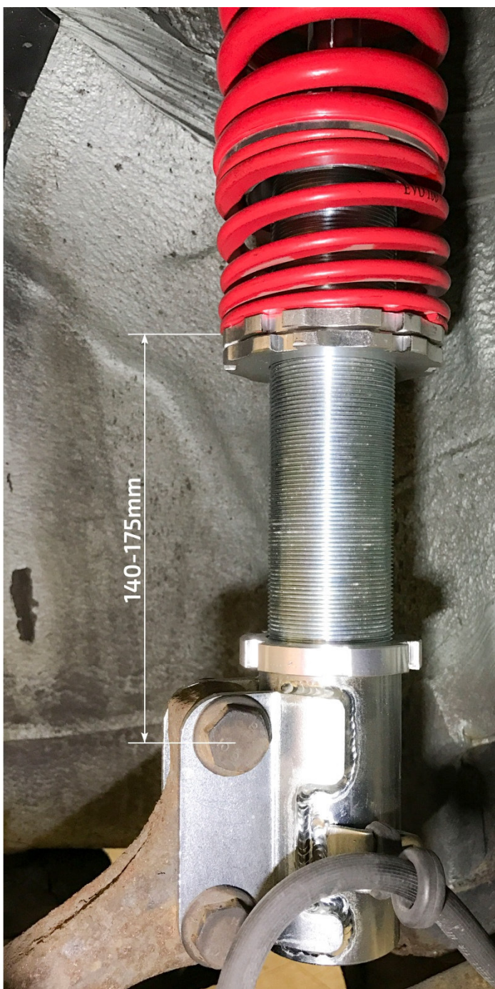
Fahrwerk Achse 1
