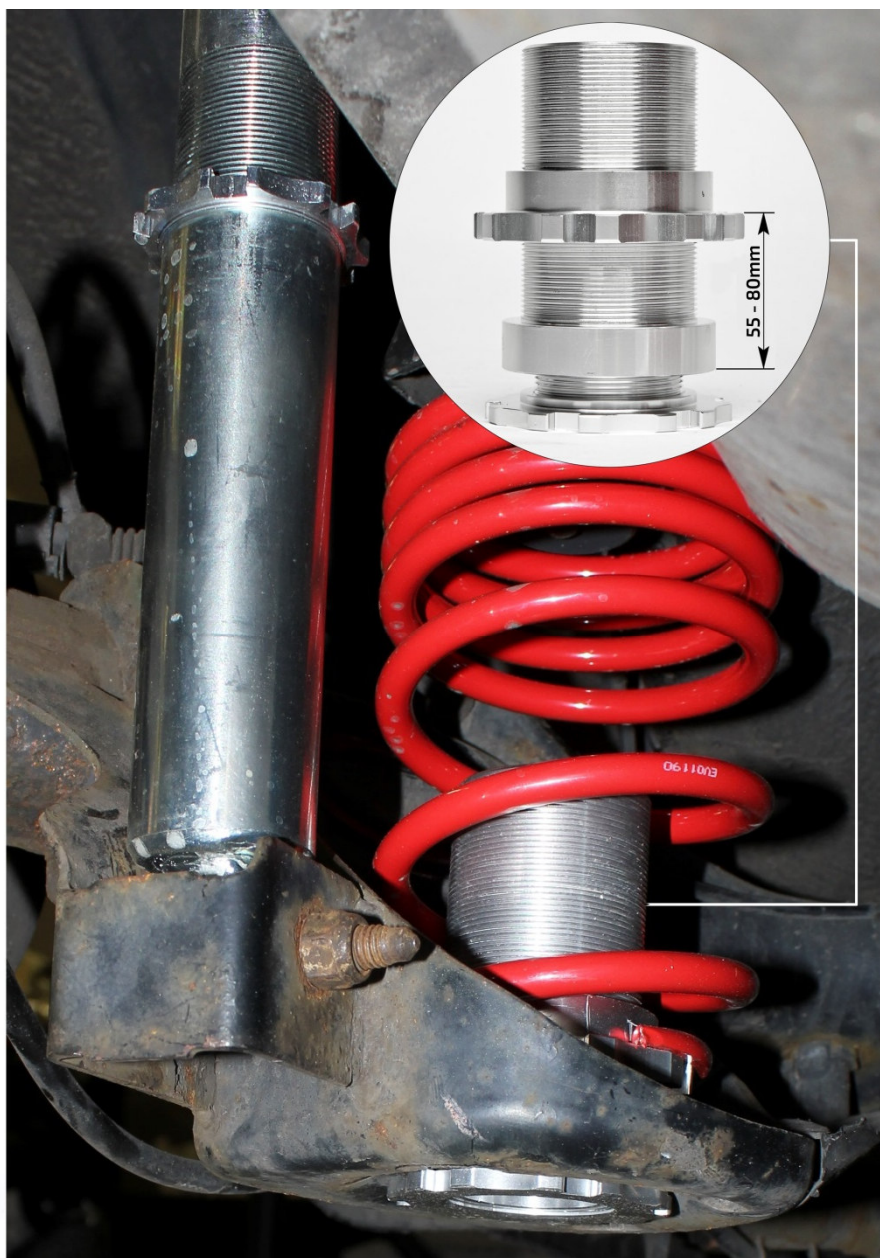
Hinterachse
