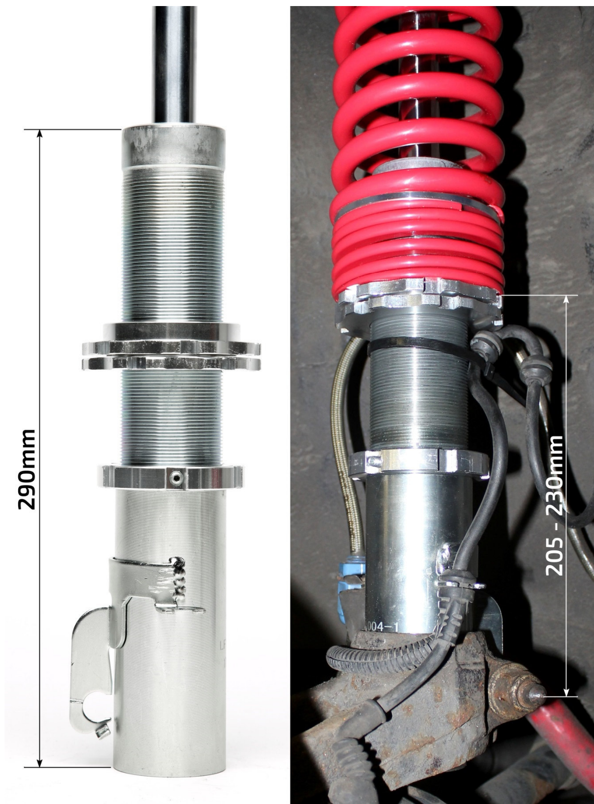
Vorderachse
